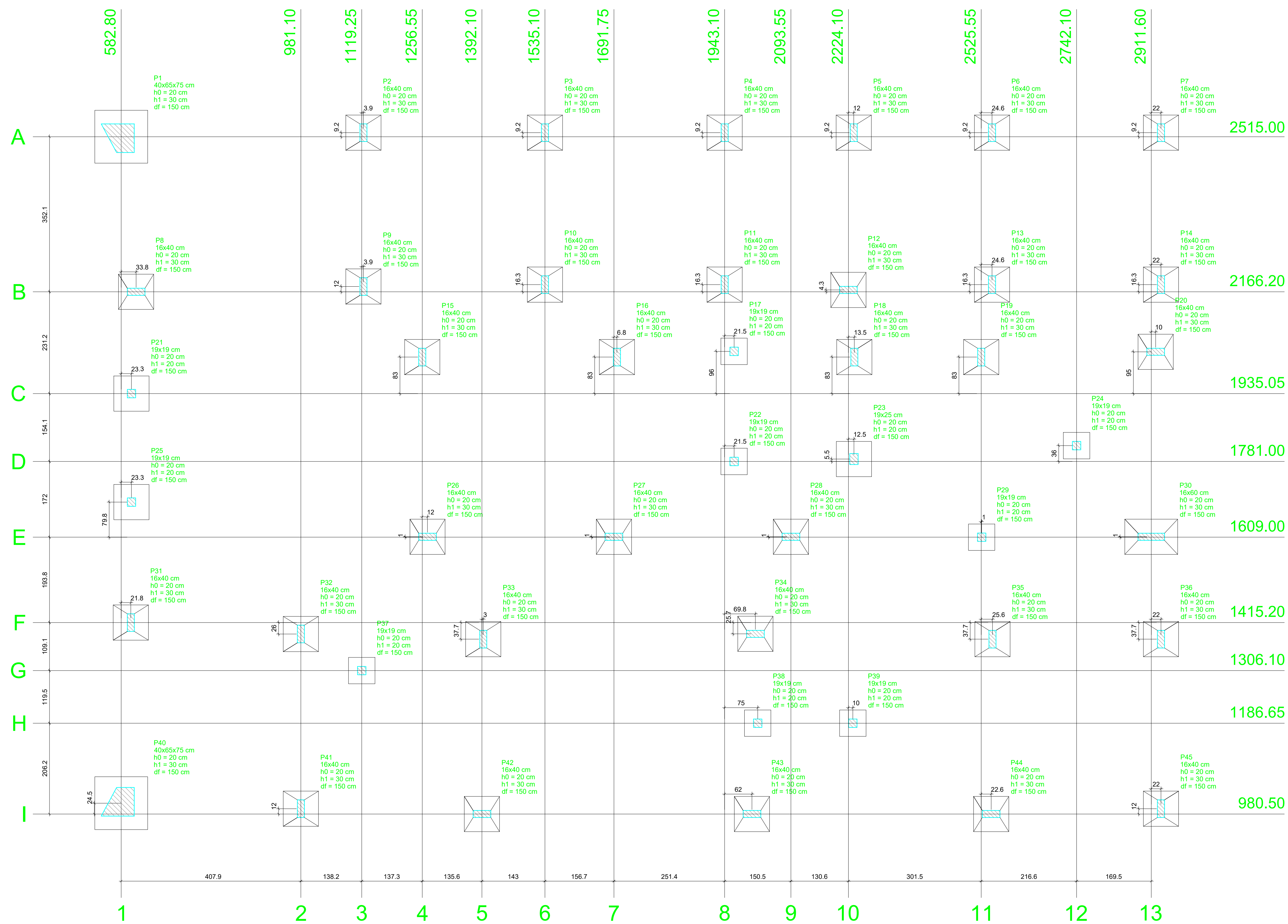
Planta de locação escala 1:50
