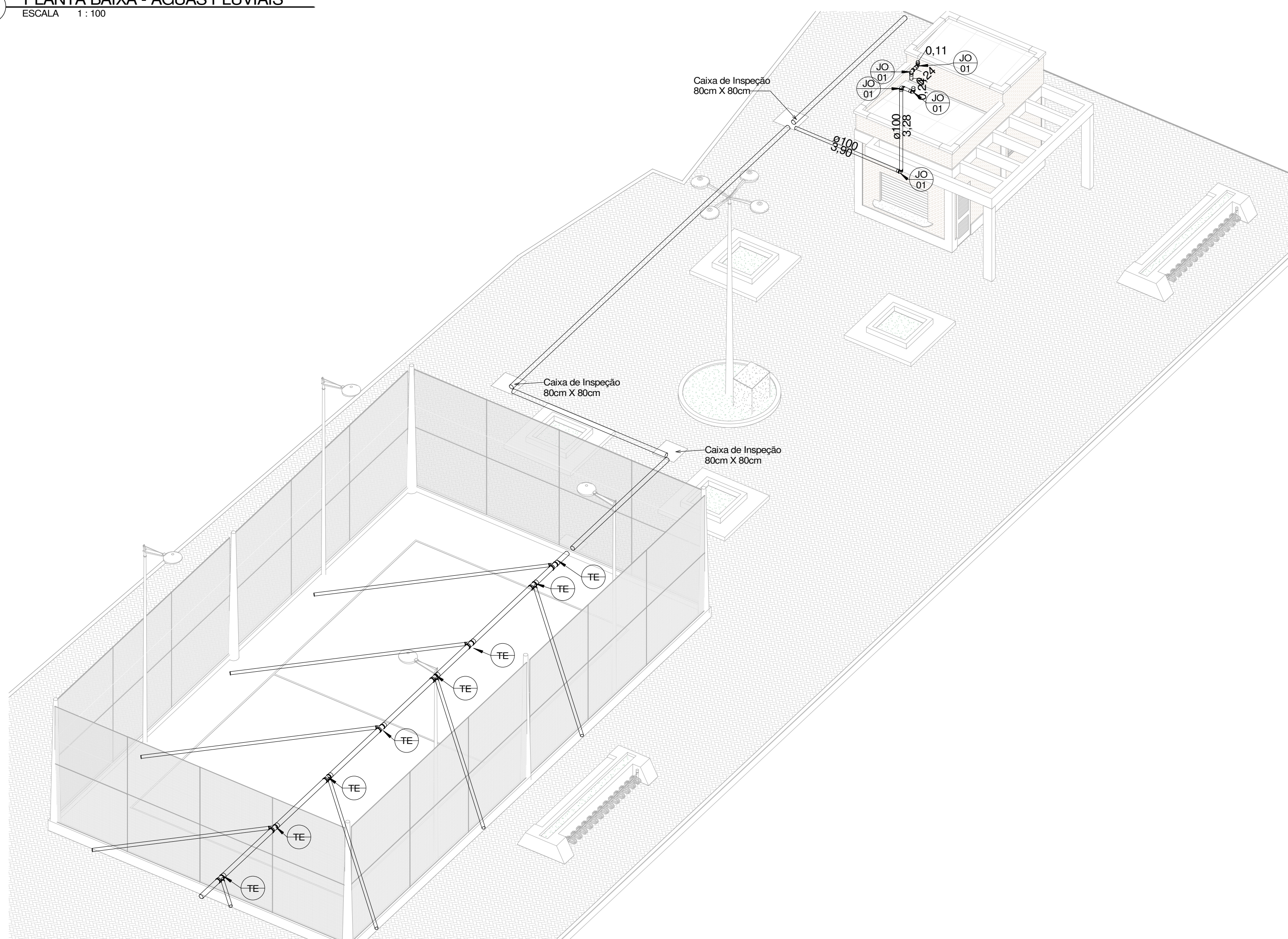
2 ISOMÉTRICO ESCALA
