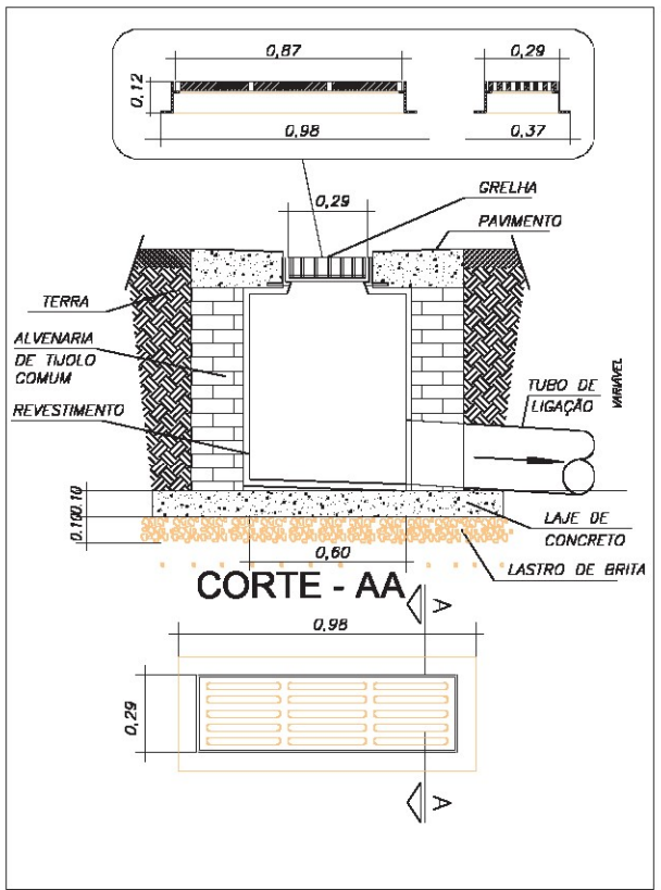
02 Detalhamento boca de leão esc. 1:25
