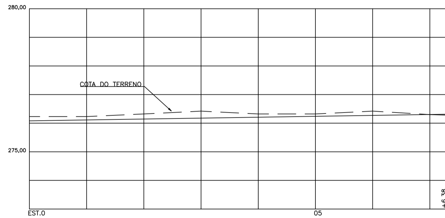
DIRETRIZ DA VIA ESCALA 1/1000
