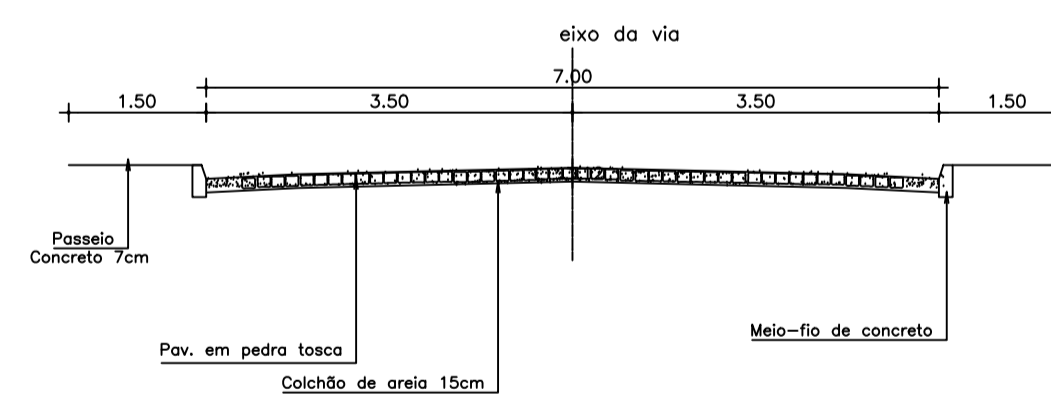
SEÇÃO TRANSVERSAL ESCALA 1/100
