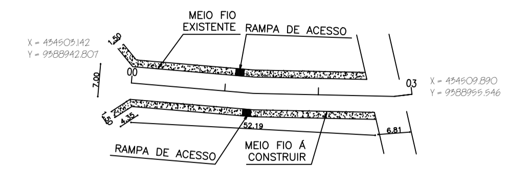
DIRETRIZ DA VIA ESCALA 1/1000
