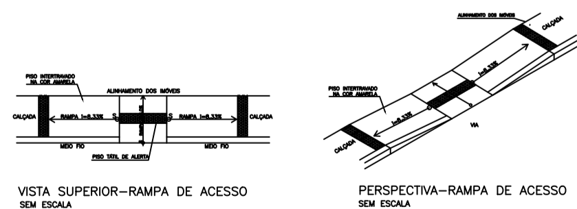
VISTA SUPERIOR-RAMPA DE ACESSO SEM ESCALA
