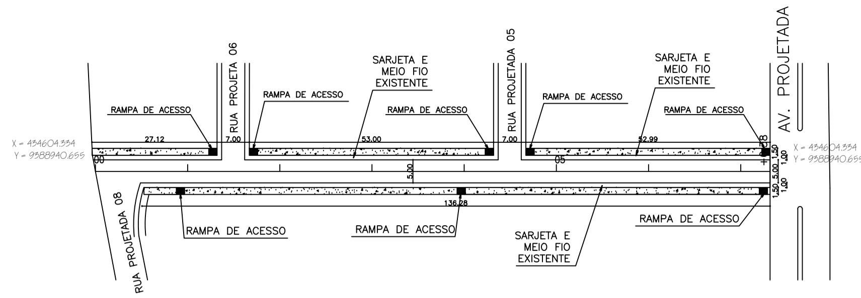
DIRETRIZ DA VIA ESCALA 1/1000
