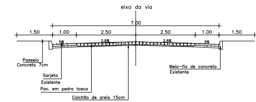
SEÇÃO TRANSVERSAL ESCALA 1/100
