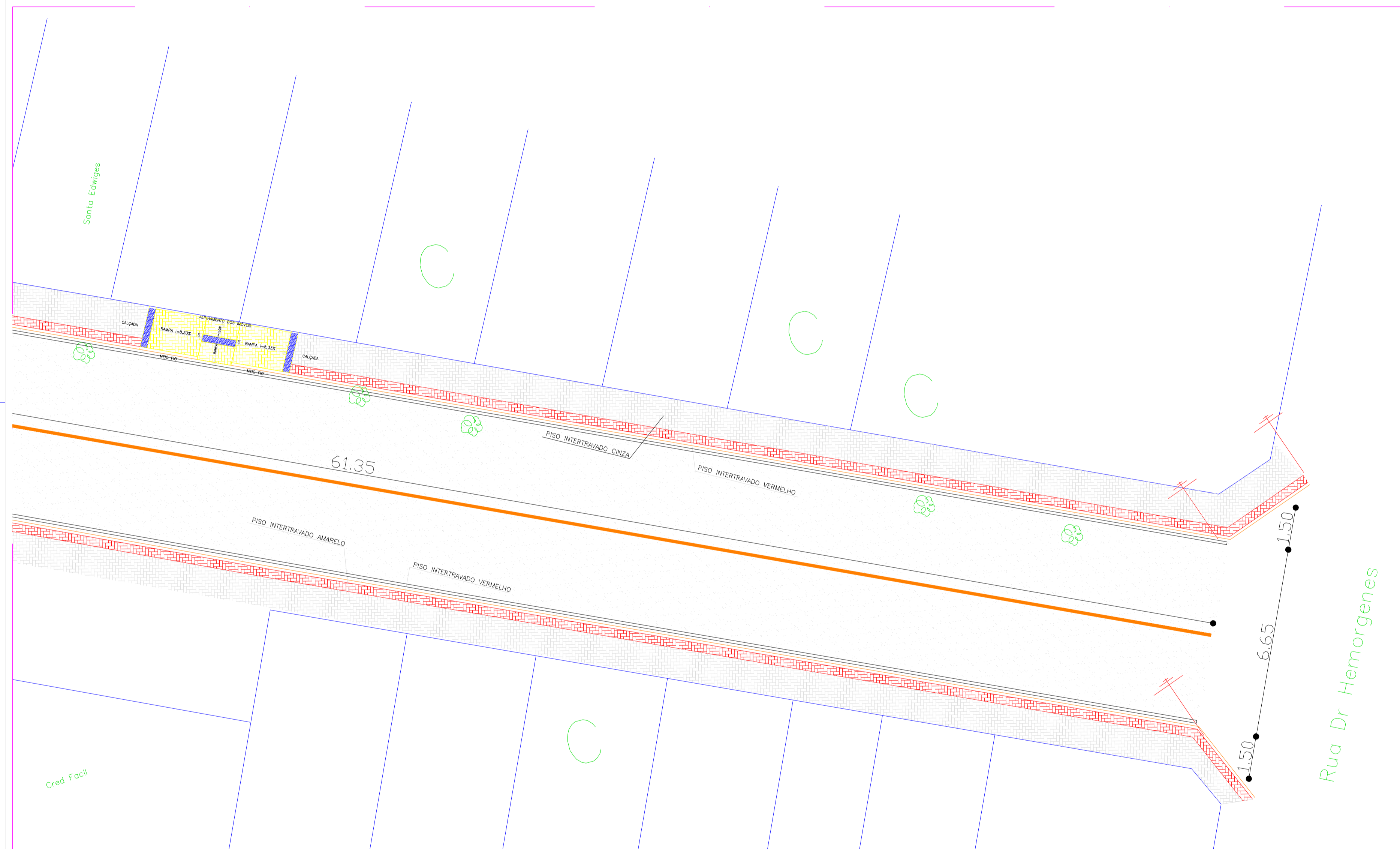
DETALHAMENTO - TRECHO 09 ESCALA 1/100
