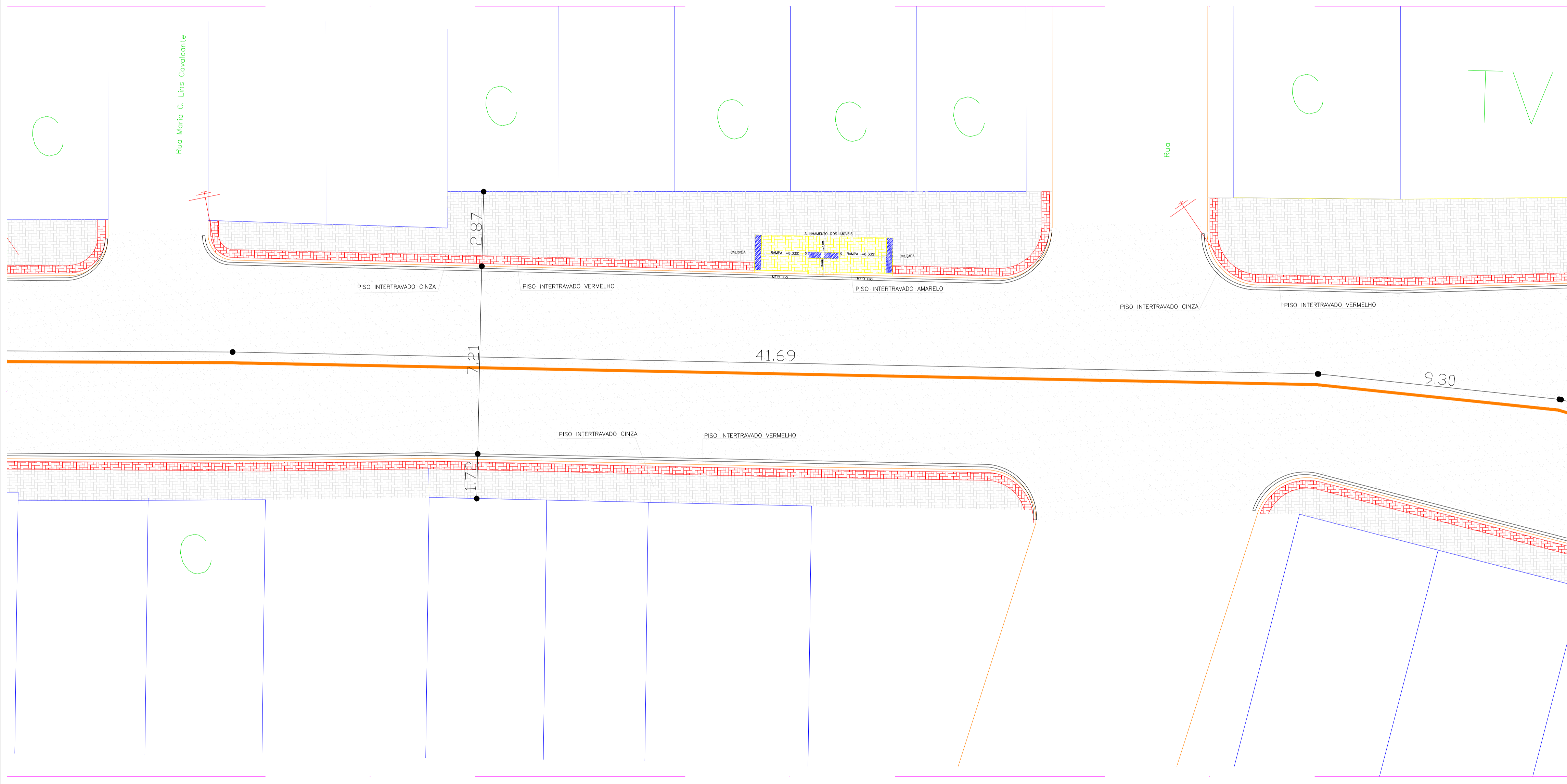
DETALHAMENTO - TRECHO 06 ESCALA 1/100
