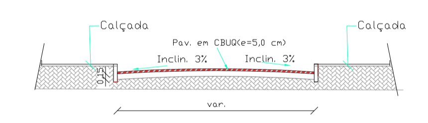
SEÇÃO TRANSVERSAL TIPO DA RUA
