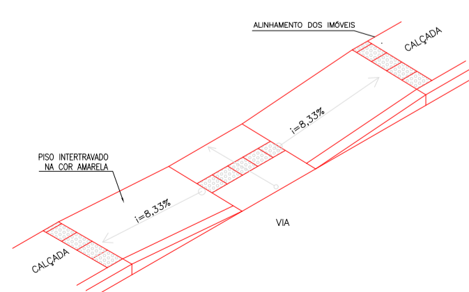
PERSPECTIVA-RAMPA DE ACESSO SEM ESCALA
