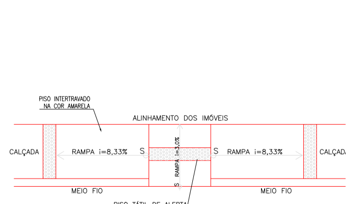
VISTA SUPERIOR-RAMPA DE ACESSO SEM ESCALA
