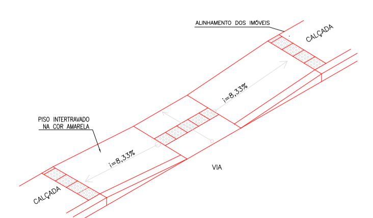
PERSPECTIVA-RAMPA DE ACESSO SEM ESCALA
