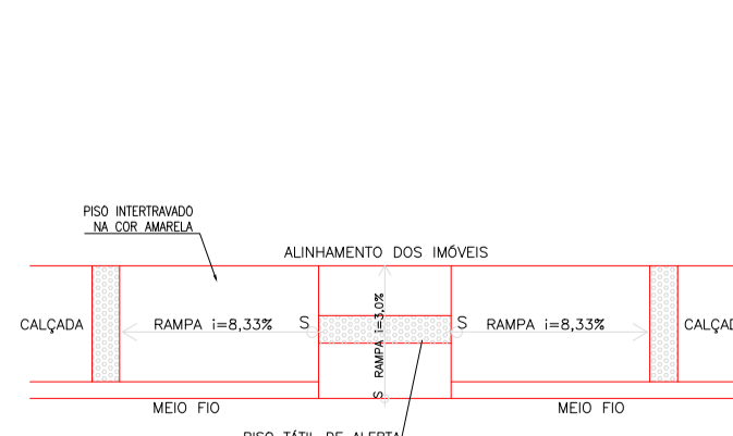
VISTA SUPERIOR-RAMPA DE ACESSO SEM ESCALA
