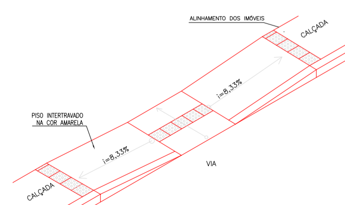
PERSPECTIVA-RAMPA DE ACESSO SEM ESCALA
