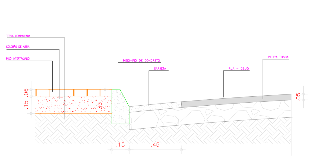
DETALHE DA PAGINAÇÃO
