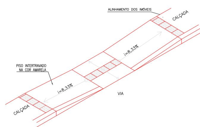
PERSPECTIVA-RAMPA DE ACESSO SEM ESCALA
