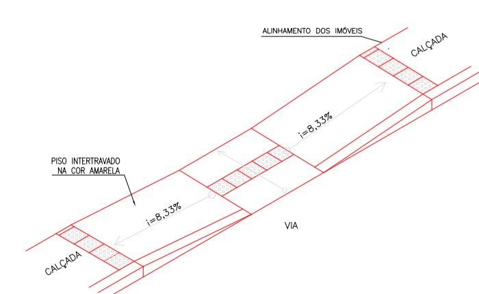
PERSPECTIVA-RAMPA DE ACESSO SEM ESCALA
