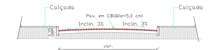
SEÇÃO TRANSVERSAL TIPO DA RUA
