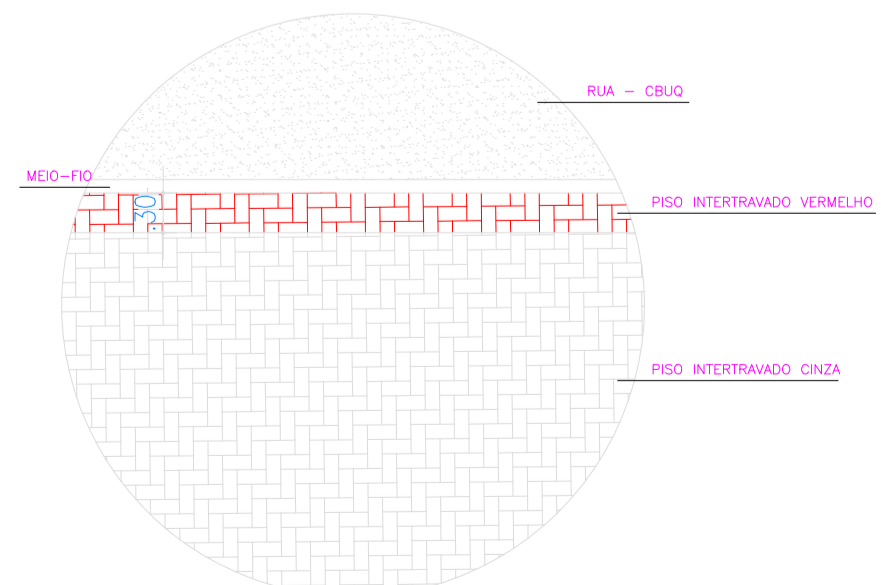
DETALHE DA PAGINAÇÃO
