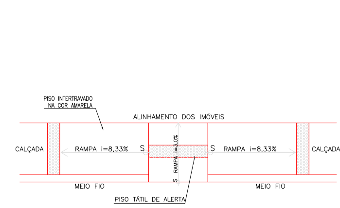
VISTA SUPERIOR-RAMPA DE ACESSO SEM ESCALA
