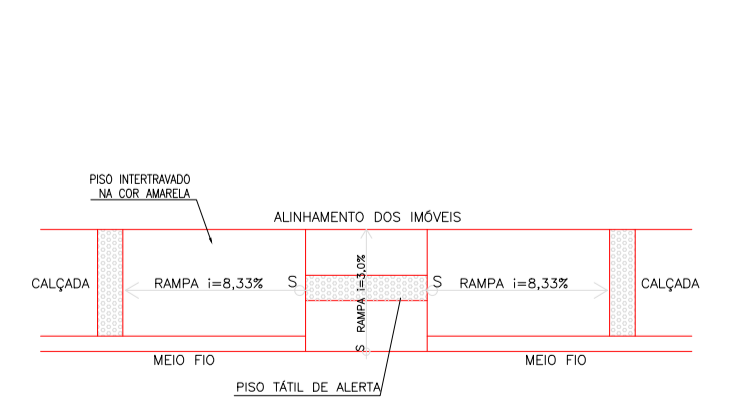
VISTA SUPERIOR-RAMPA DE ACESSO SEM ESCALA
