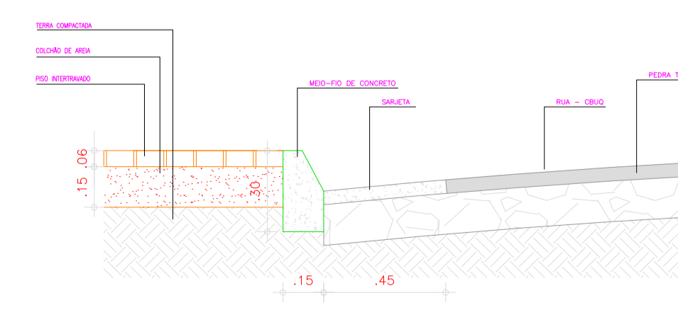
DETALHE DA PAGINAÇÃO
