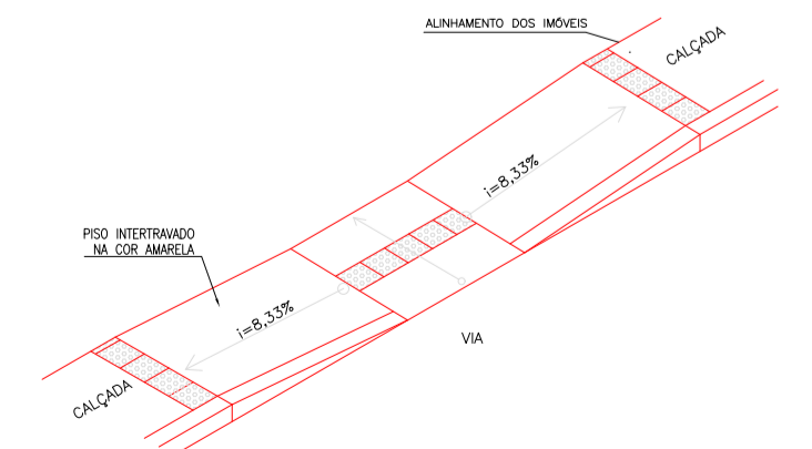
PERSPECTIVA-RAMPA DE ACESSO SEM ESCALA
