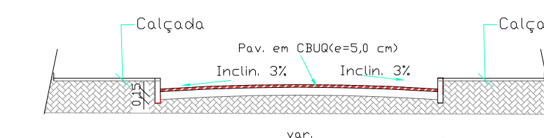
SEÇÃO TRANSVERSAL TIPO DA RUA
