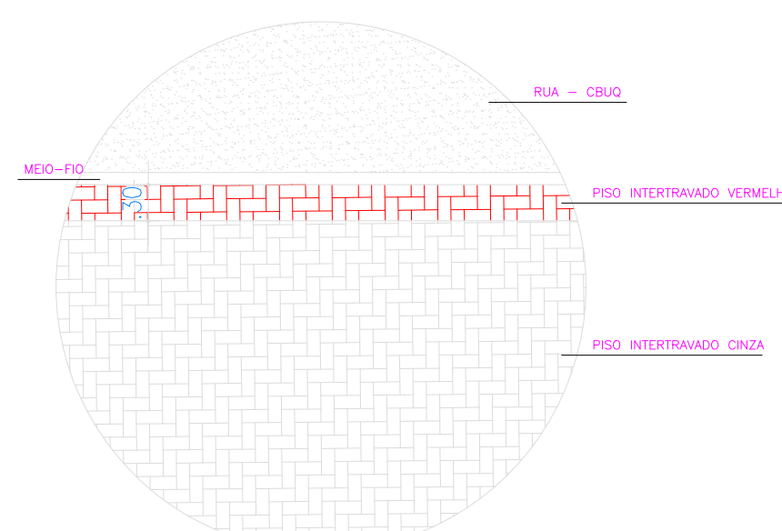
DETALHE DA PAGINAÇÃO
