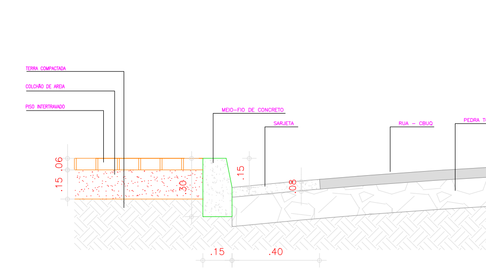
DETALHE DA PAGINAÇÃO
