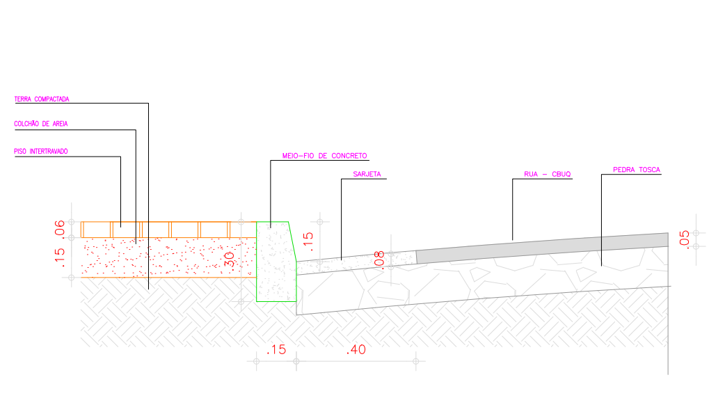
DETALHE DA PAGINAÇÃO
