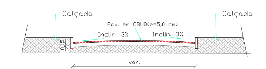
SEÇÃO TRANSVERSAL TIPO DA RUA
