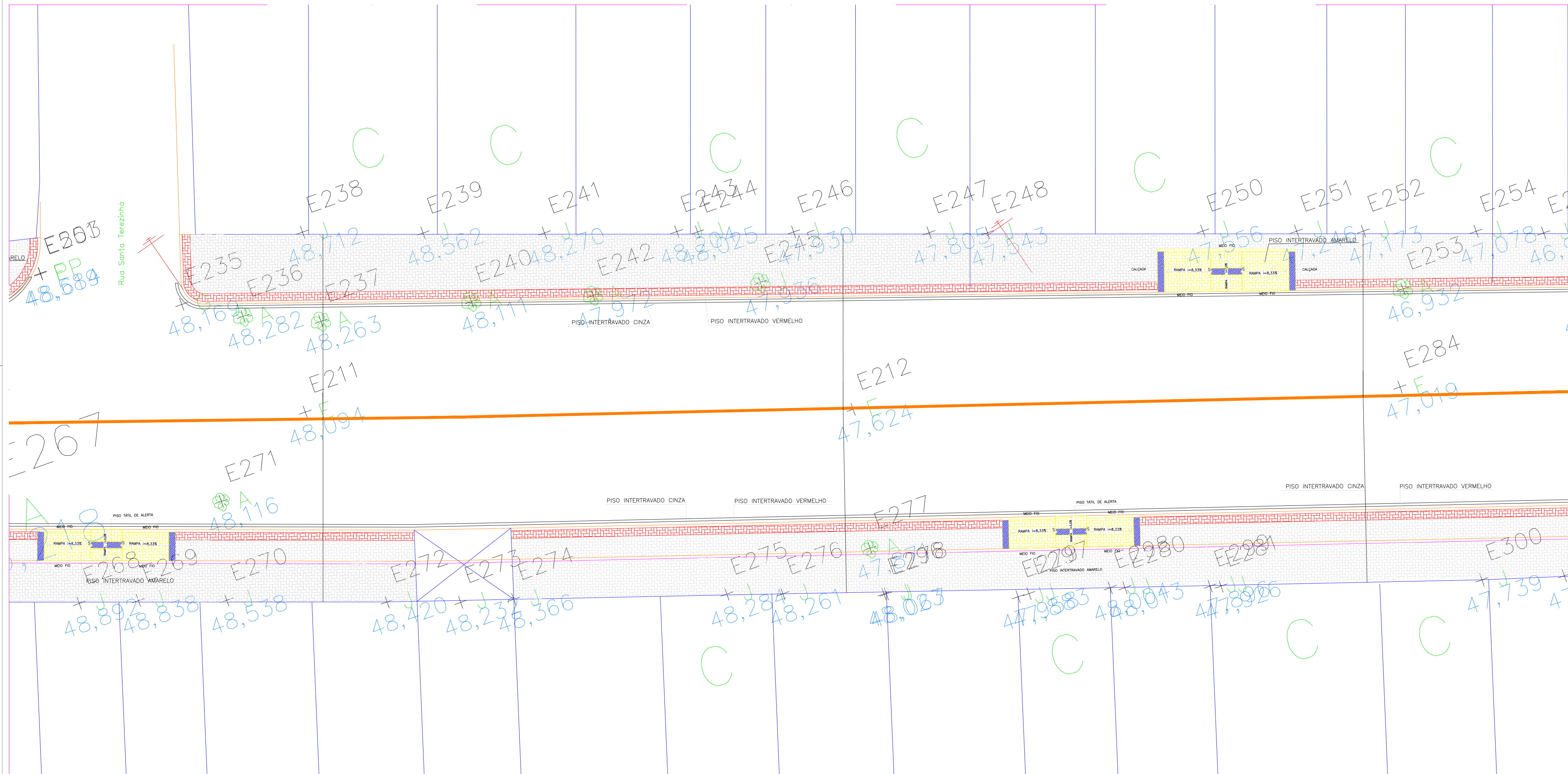
DETALHAMENTO - TRECHO 03 ESCALA 1/100
