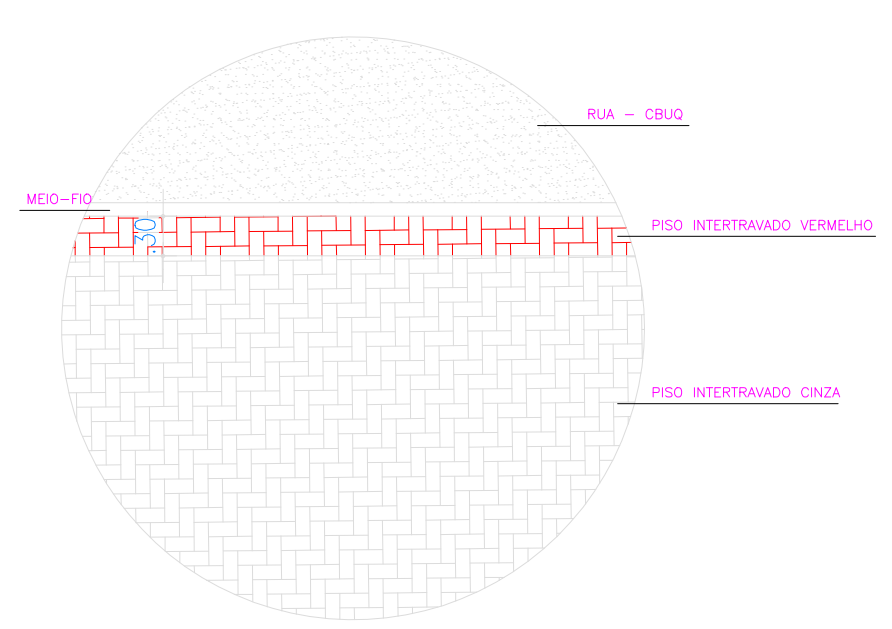
DETALHE DA PAGINAÇÃO
