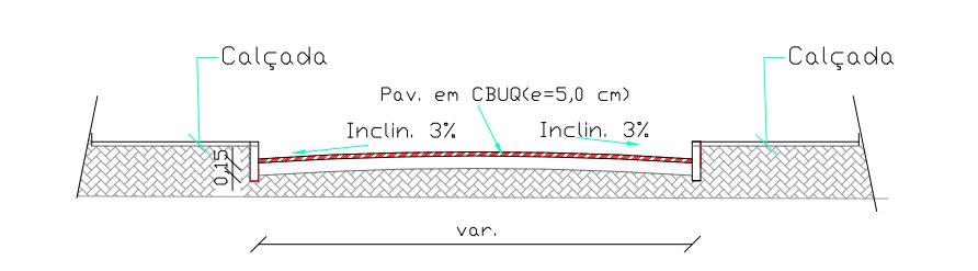
SEÇÃO TRANSVERSAL TIPO DA RUA
