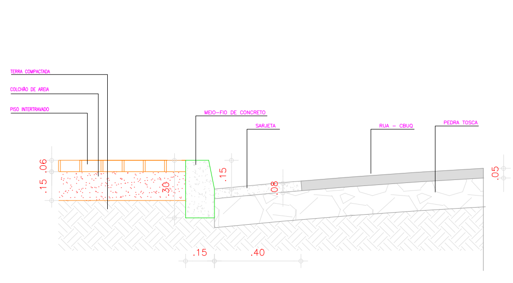
DETALHE DA PAGINAÇÃO
