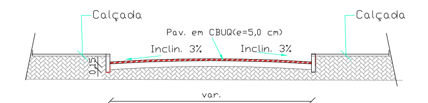
SEÇÃO TRANSVERSAL TIPO DA RUA
