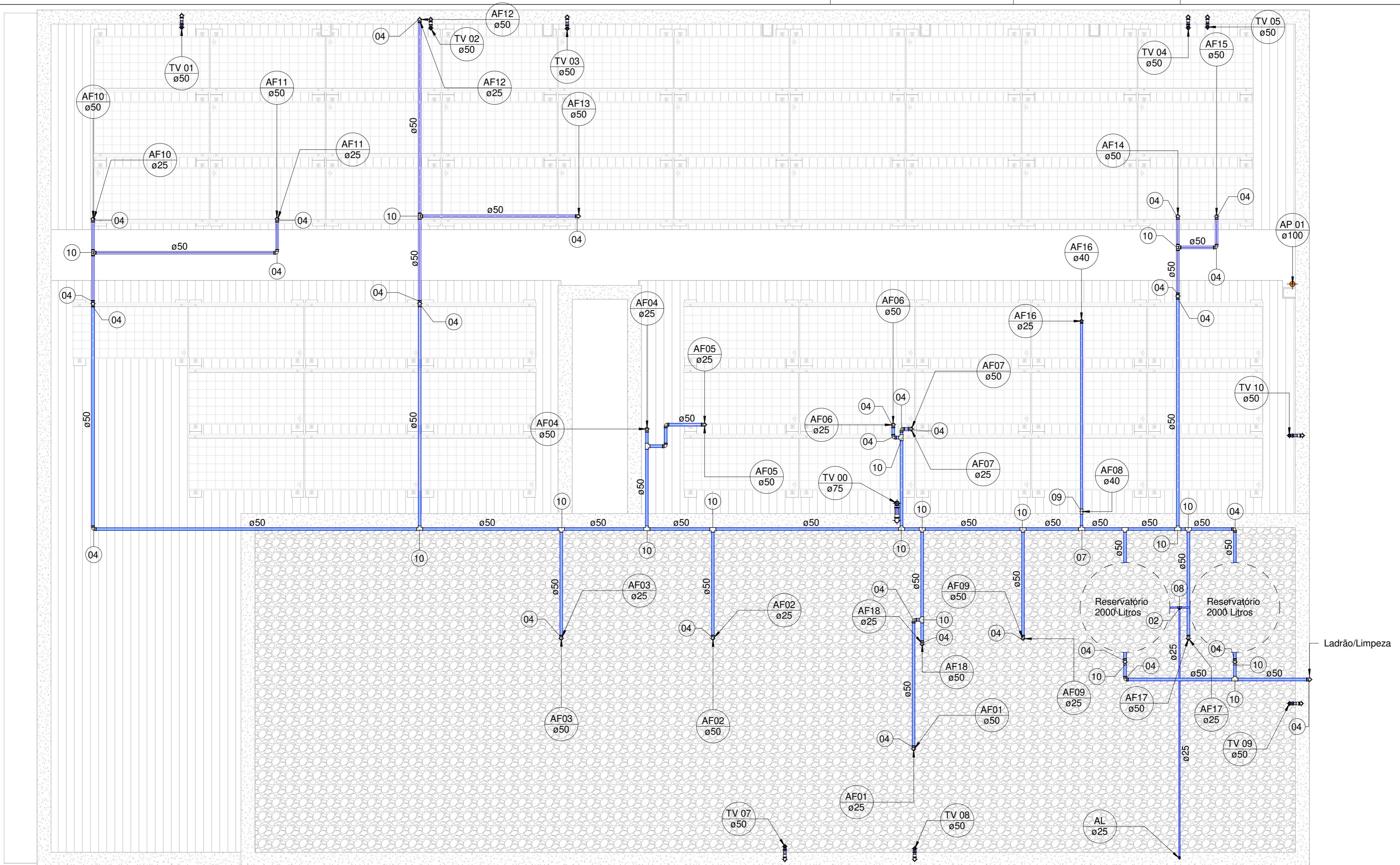
1 Planta Chave - Cobertura 1 : 50
