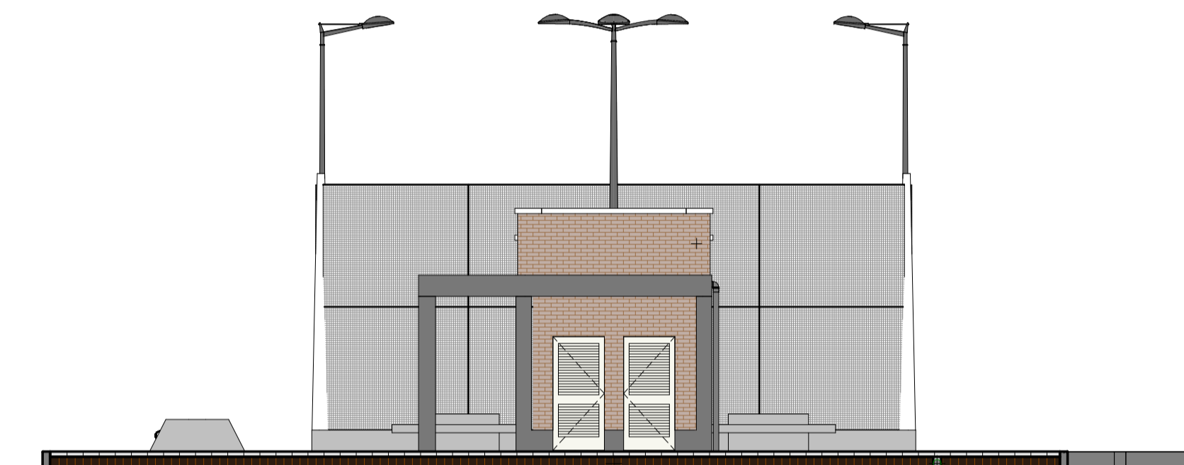
2 CORTE B-B ESCALA 1:100
