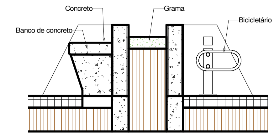
3 CORTE G-G ESCALA 1:20
