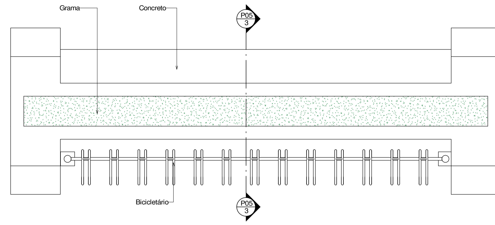
2 BANCO BICICLETÁRIO ESCALA 1:25
