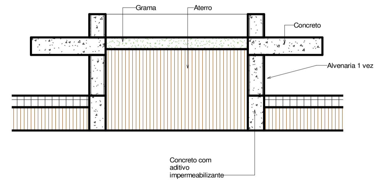
6 CORTE F-F ESCALA 1:20
