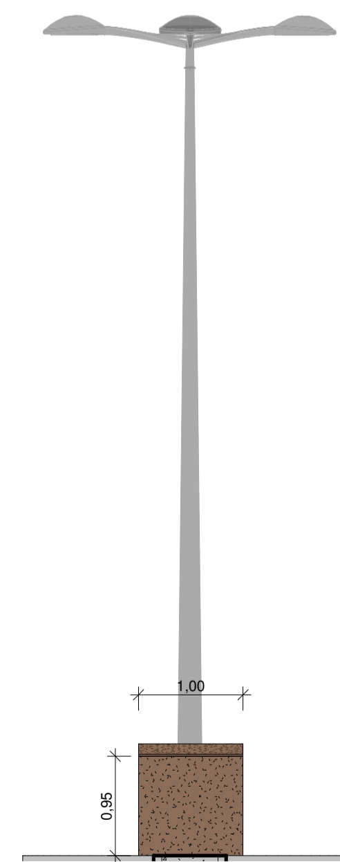
8 CORTE H-H ESCALA 1:50
