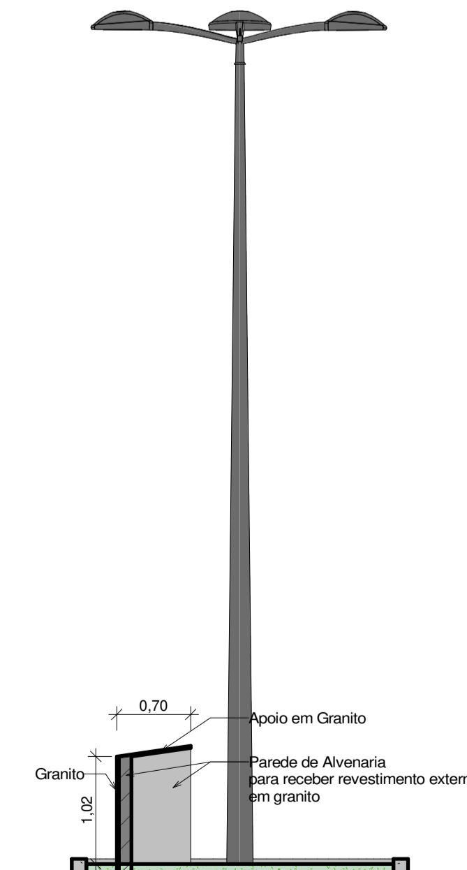
9 CORTE I-I ESCALA 1:50
