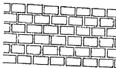
AJUSTE CORRENTE (um tijolo)
