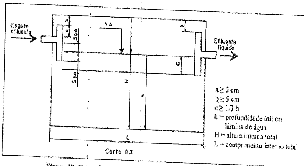
Figura 12. Corte de um tanque séptico (NBR 7229/93, Anexo A, figura 3)
