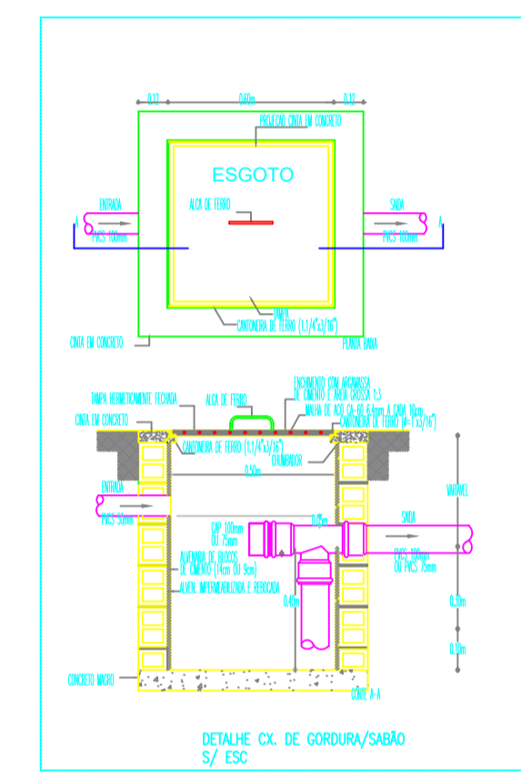
01 PLANTA DE CI, CG E CP ESCALA 1/25
