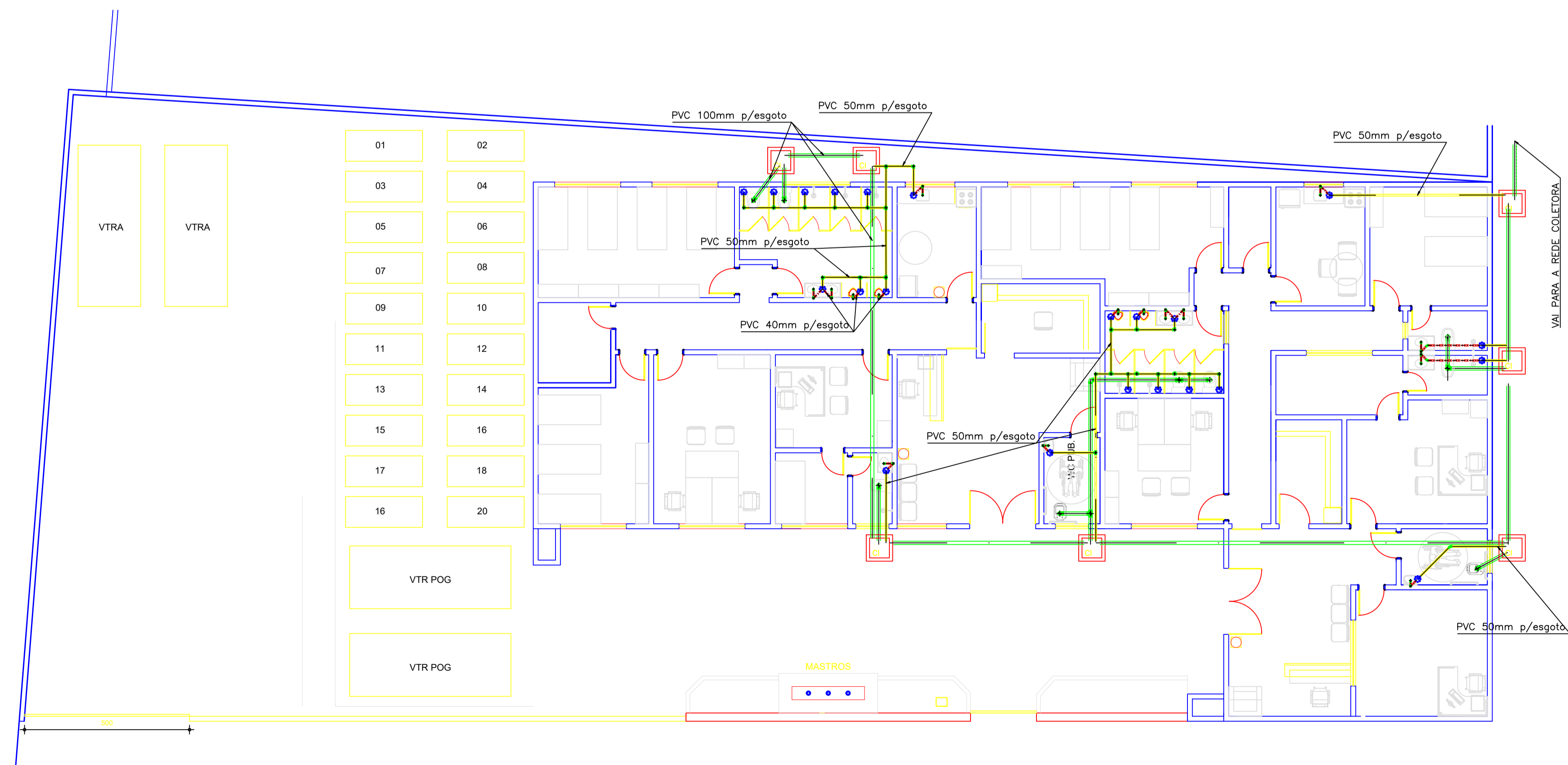
02 PLANTA SANITÁRIA ESCALA 1/100
