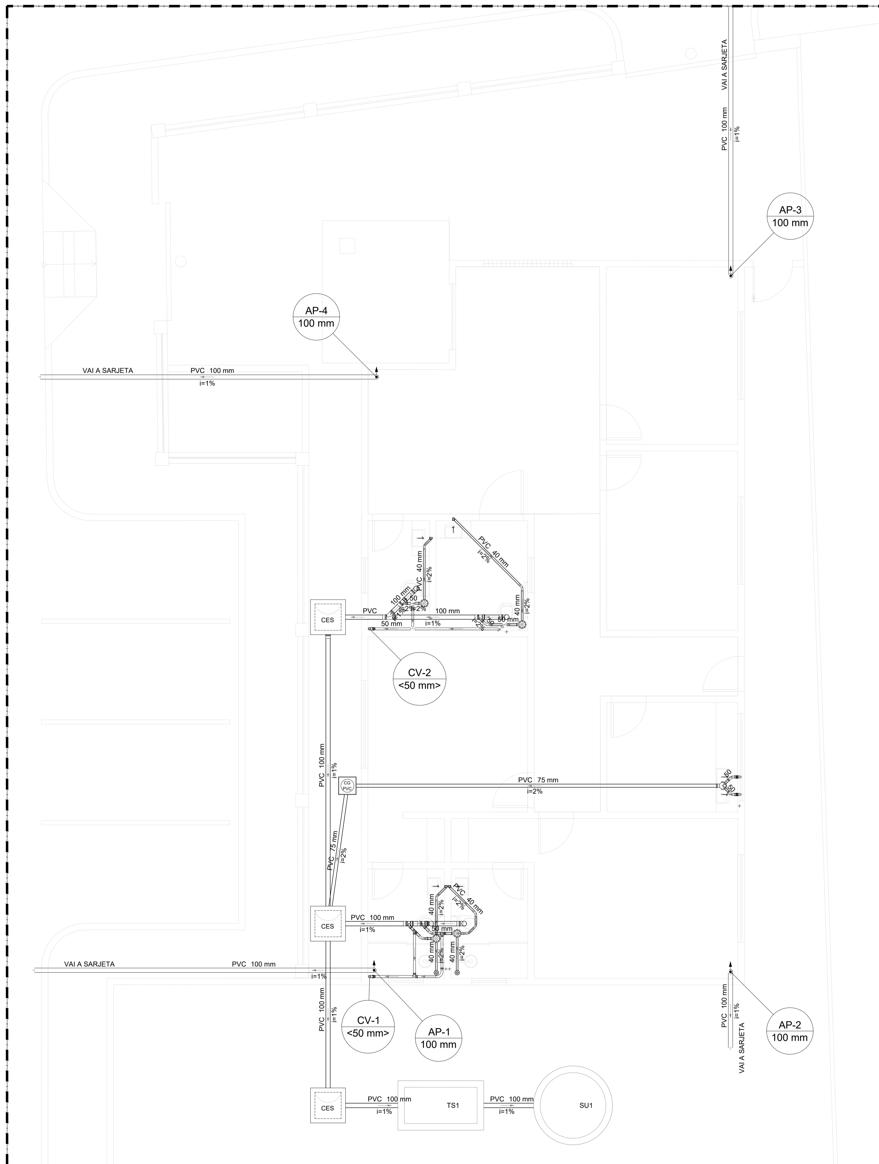
11.00 PLANTA BAIXA - SANITÁRIO ESCALA 1/50
